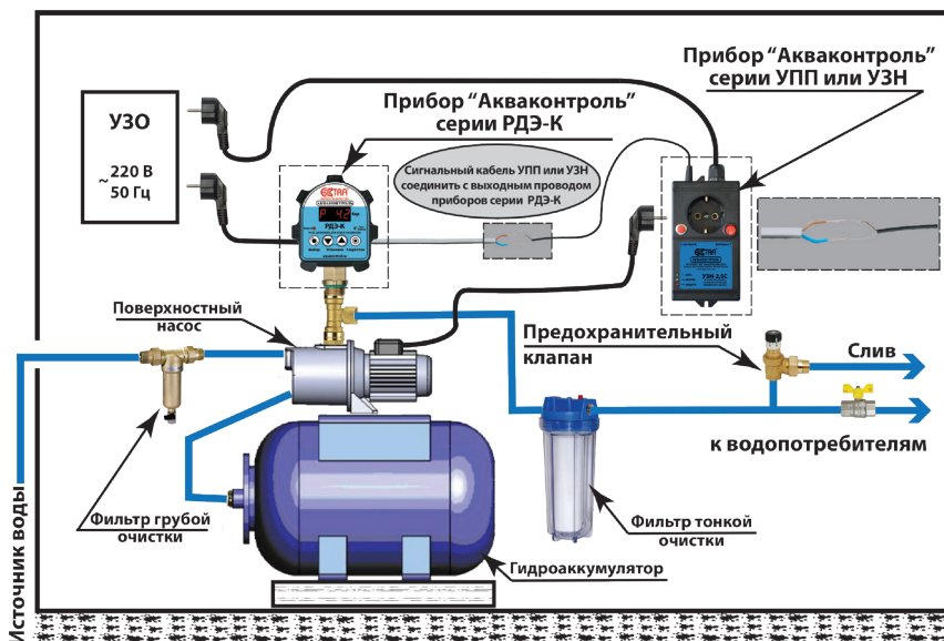
Пример 6. Подключение РДЭ-К к УПП или УЗН "Extra Акваконтроль" без использования адаптера АПП.
