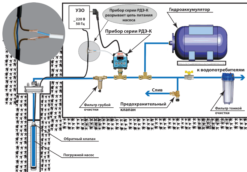
Пример 6. Подключение РДЭ-К к УПП или УЗН "Extra Акваконтроль" без использования адаптера АПП.
