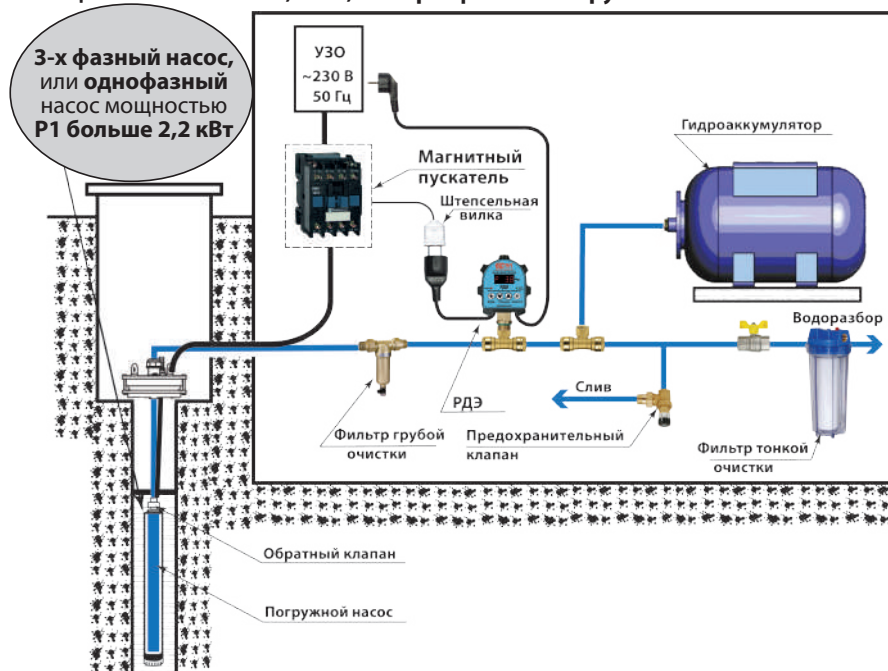
Пример 4. Подключение РДЭ для управления однофазным насосом мощностью Р1 более 2,2 кВт, или трехфазным погружным насосом.
