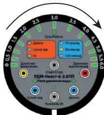
Верное включение светодиодов
